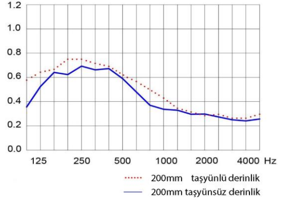
EN ISO 354 ses yutum katsayısı ölçümü
